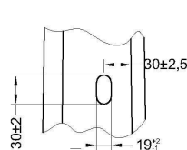
DETALHE A
