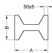
DETALHE C
